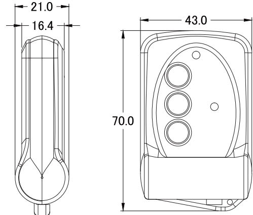
左視圖
