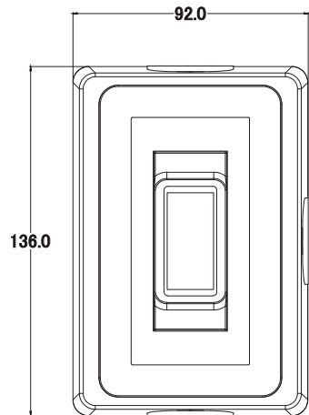
前視圖
