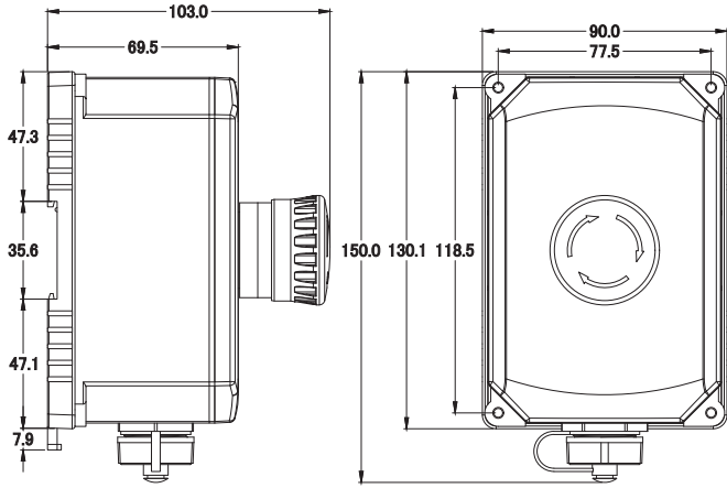
左視圖
